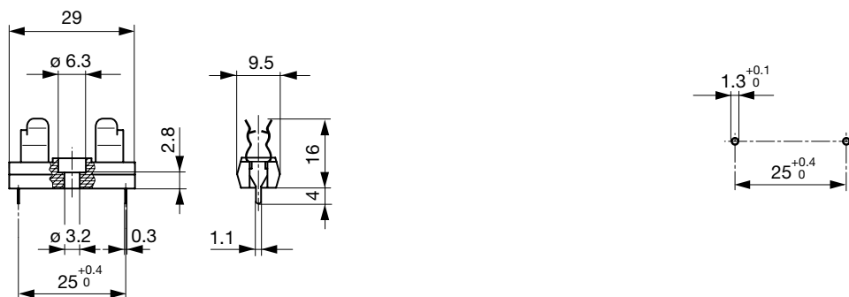
Bohrplan
