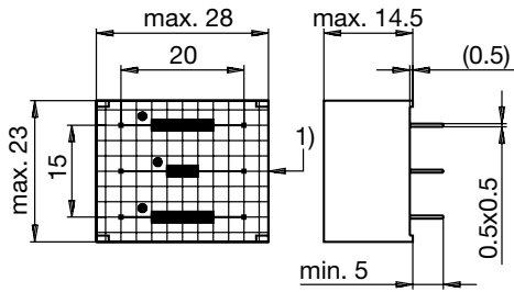
Gehäuse 05-7
