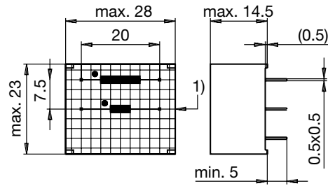
Gehäuse 05-8
