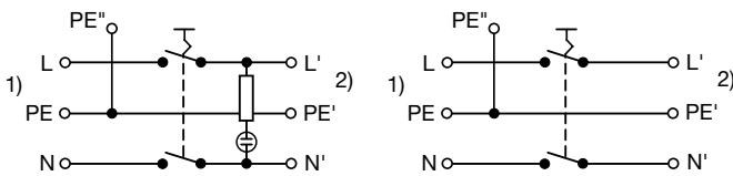
1) Netz 2) Last
