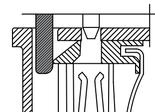
Verriegelungsvorgang: entriegelt (offen) beim Einstecken des Steckers
