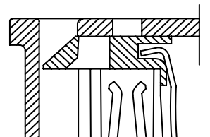
Verriegelungsvorgang: verriegelt (geschlossen), nach dem Entfernen des Steckers
