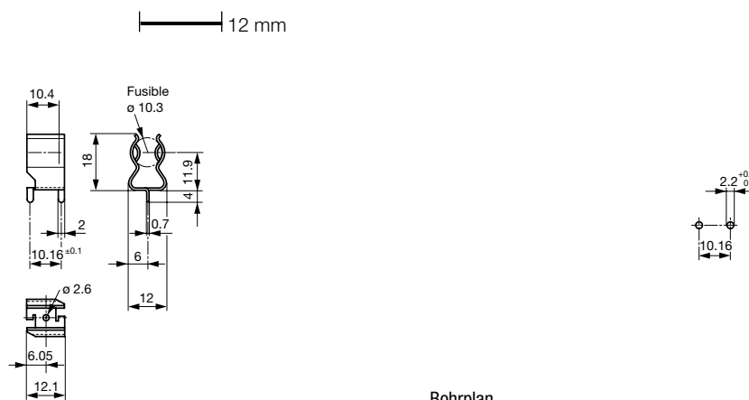
Bohrplan
